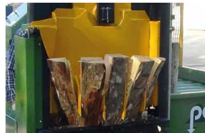
Cuneo con 4 coltelli orbitali per ottenere 5 ceppi a ciclo
